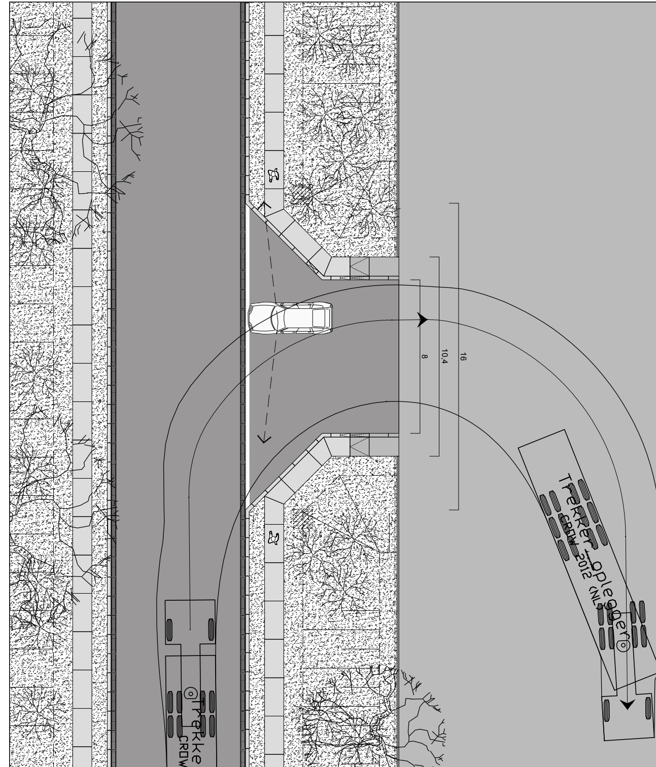
inrit bedrijfskavel: 8m (24m aan de bedrijfslaan) voertuig: trekker-opleggercombinatie volgens CROW
