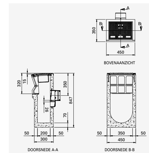
trottoirkolk passend bij Amstelband: TBS type TRK-5717
