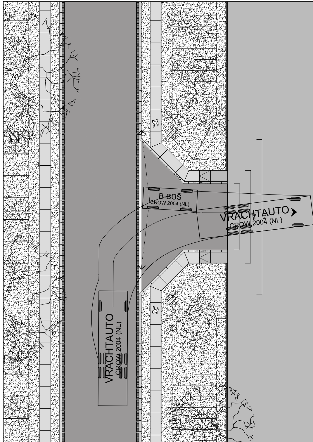
inrit bedrijfskavel: 6m (14m aan de bedrijfslaan) voertuig: ongelede vrachtwagen volgens CROW
